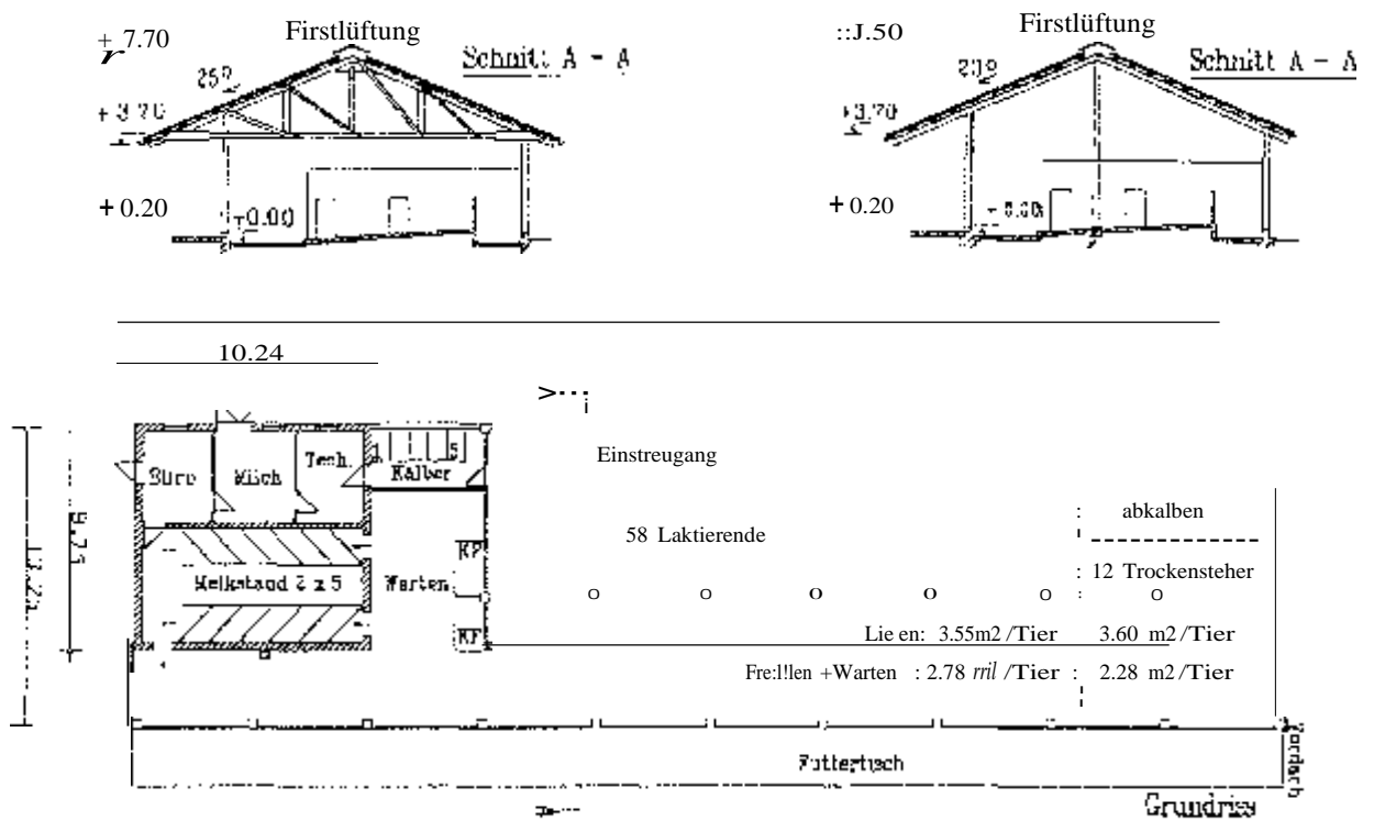
3: Tretmiststall für 70 Kühe ohne Jungvieh
