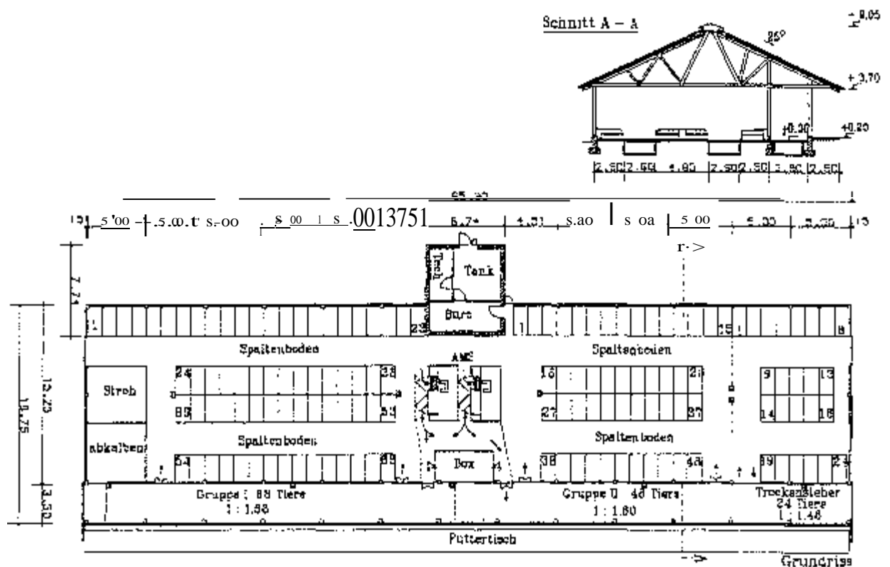
7: 4reihiger Boxenlaufstall mit zwei Einboxenanlagen
