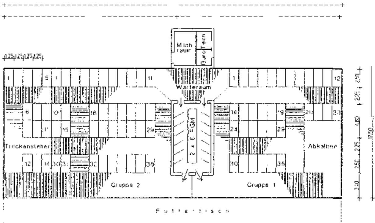
Abb. 8: 4-reiniger Liegeboxenstall mit zentraler Anordnung des Melkstandes
