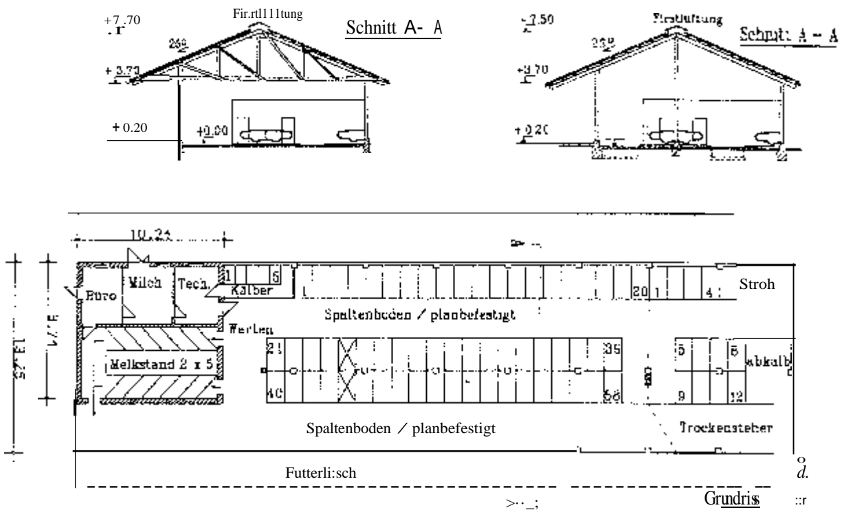
4: Offenfrontstall mit 3 Liegeboxenreihen für 70 Kühe ohne Jungvieh
