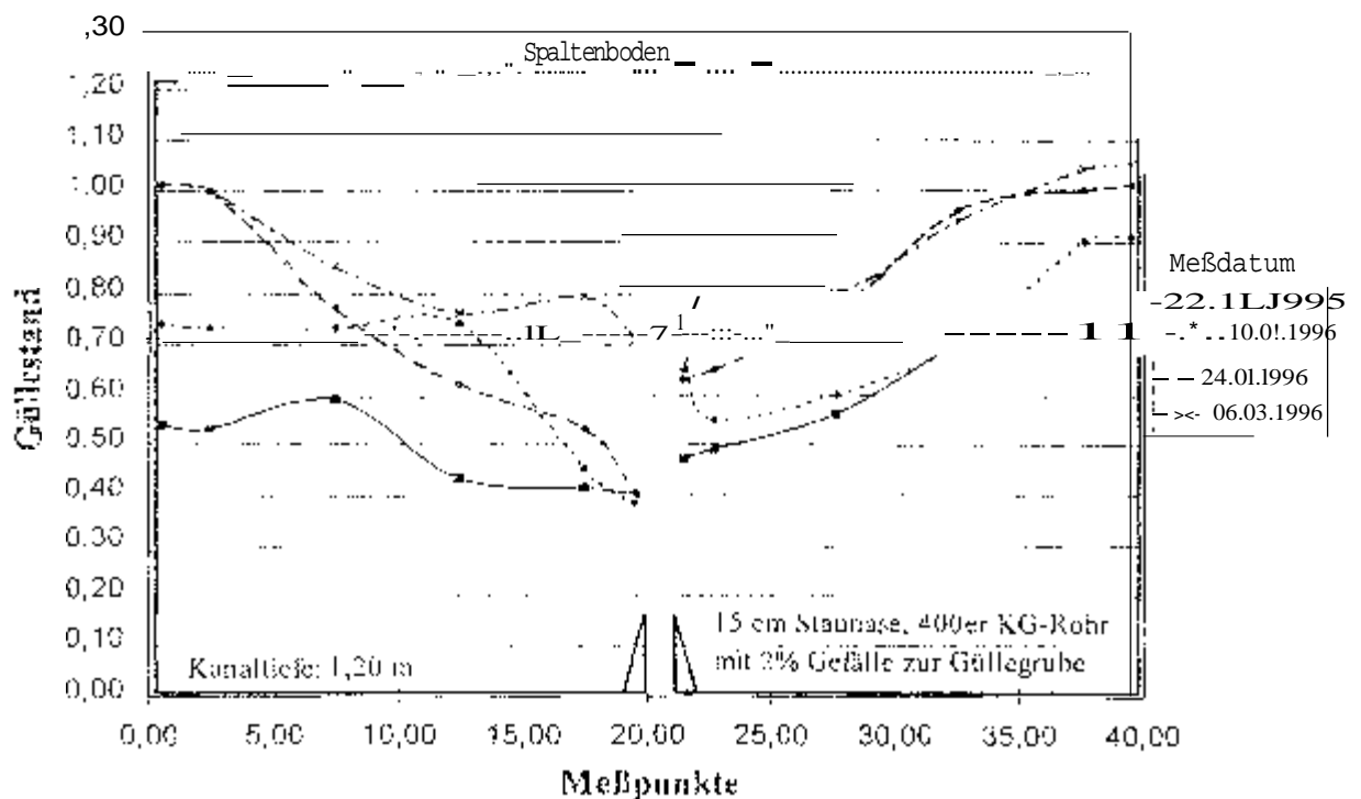
2: Güllestandsmessungen im Treibmistkanal (Winter 1995/96; Jungvieh)
