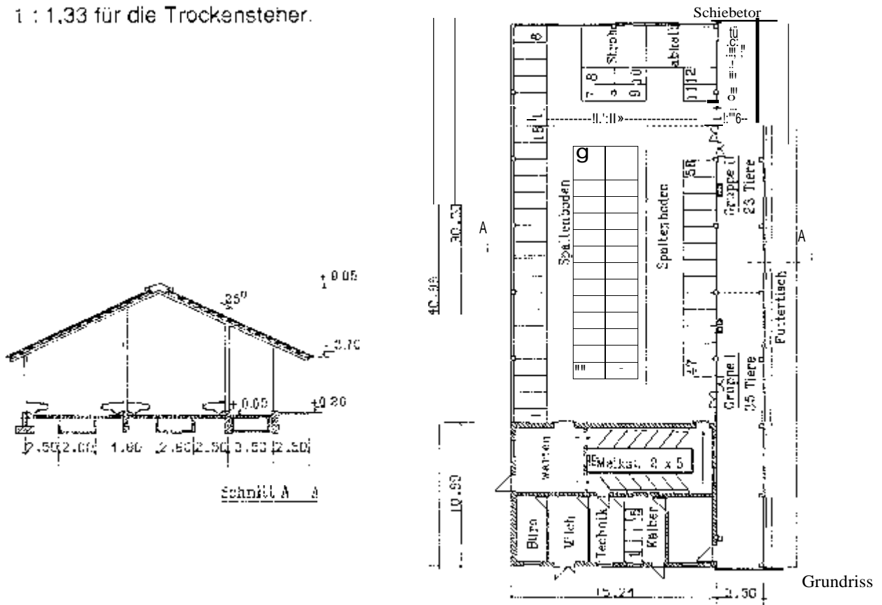
6: Vierreihiger Liegeboxenlaufstall für 70 Kühe mit Gruppenfütterung ohne Jungvieh
