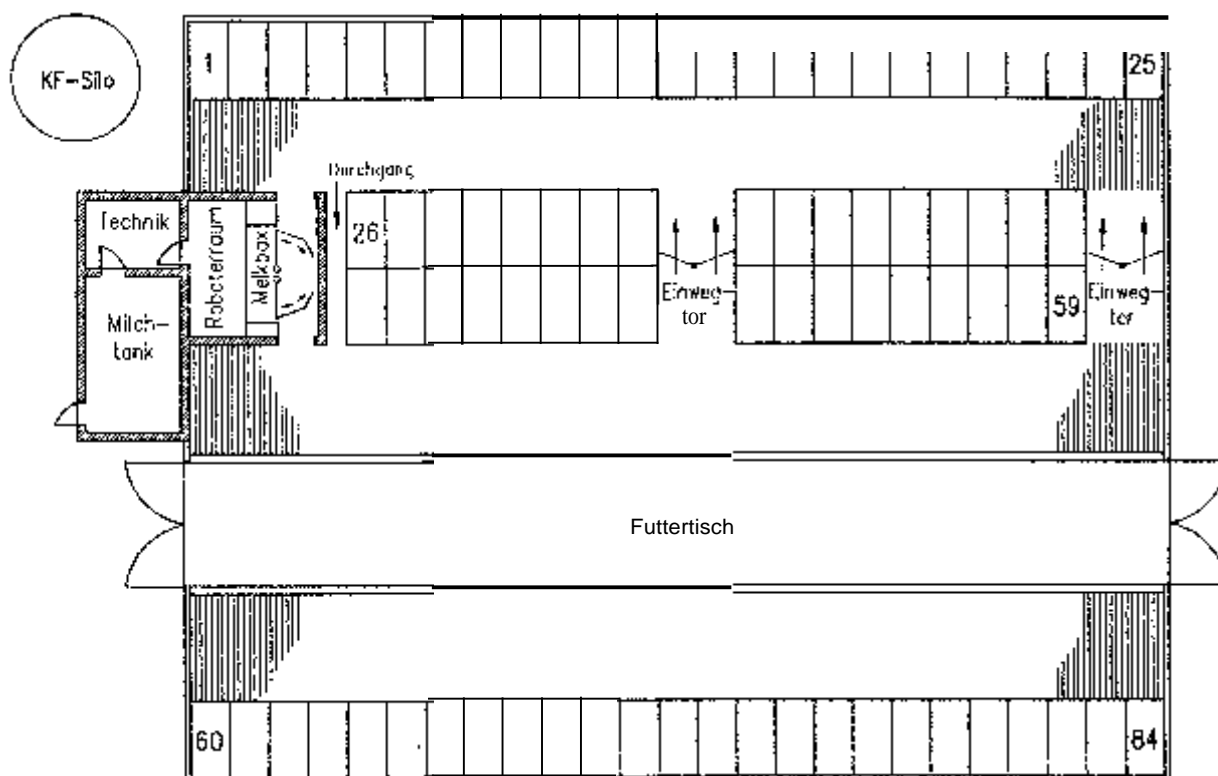
1: Liegeboxenlaufstall mit automatischem Melksystem
