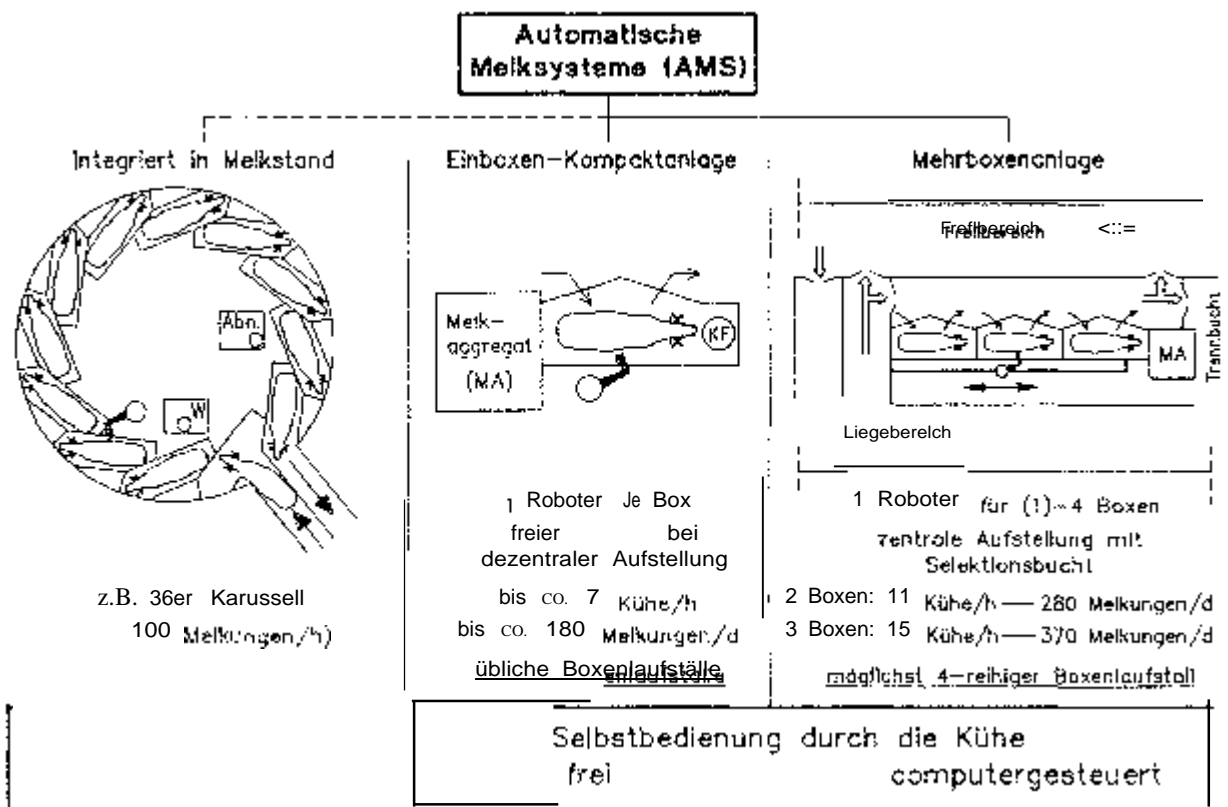
Abb. 4 Bauformen automatischer Melksysteme
