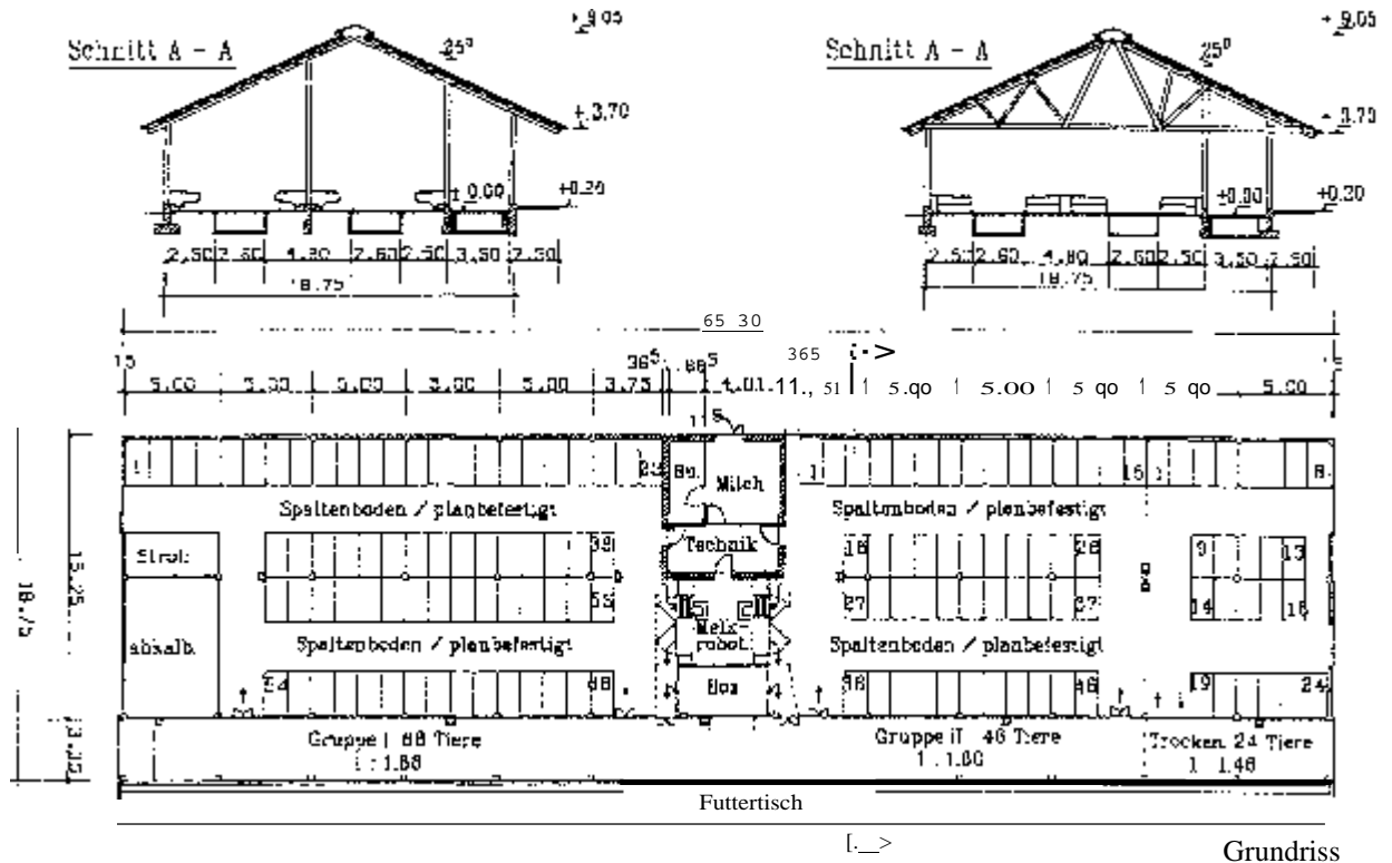
9: Vierreihiger Liegeboxenlaufstall AMS 40 Kühe Gruppenfütterung und 1
