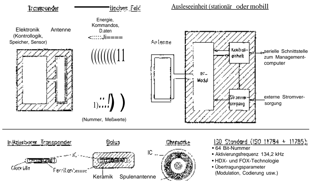
Abb. 1 Schematischer Aufbau und Systemparameter der elektronischen Kennzeichnung
