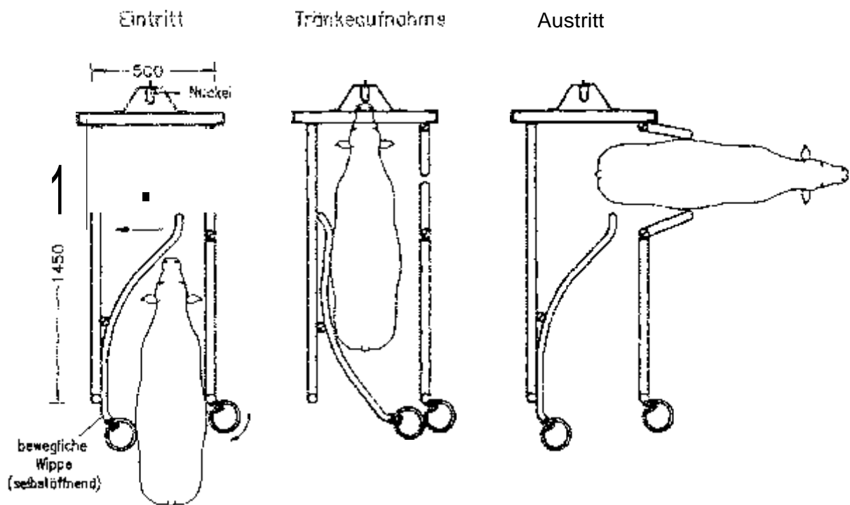
1: Schema eines verschließbaren Standes für Kälbertränkeautomaten
