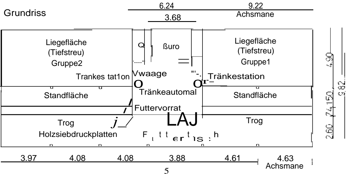
Offenfrontstall für die Fresseraufzucht mit zwei Versuchsgruppen und einem wärmeisolierten Zentralraum für die Versuchsdurchführung
