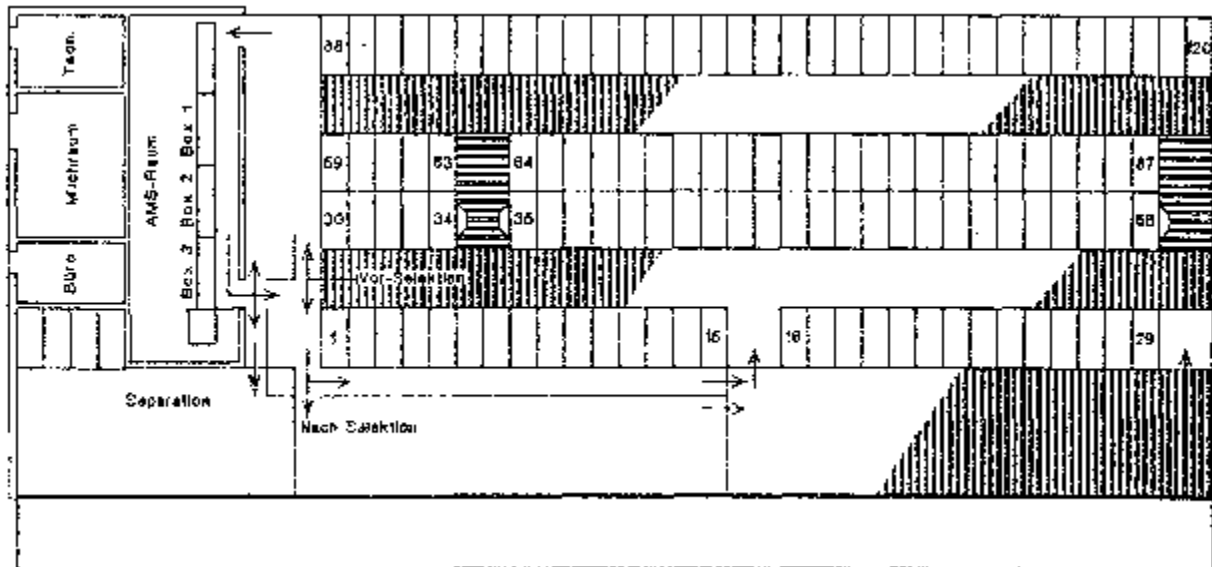
8: 4reihiger Liegeboxenlaufstall mit AMS und Gruppeneinteilung am Futtertisch (Mehrboxenanlage)
