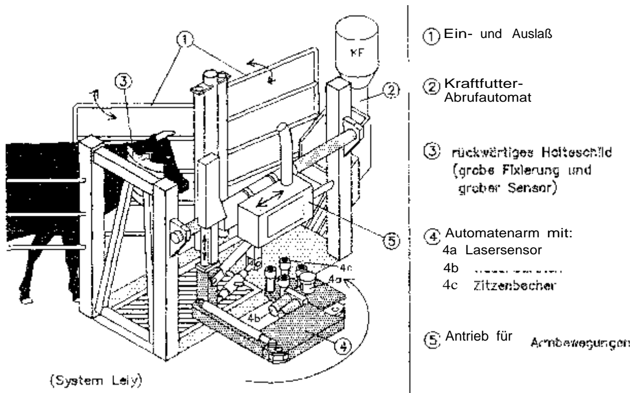
3: Funktion eines automatischen Melksystems (System Lely)
