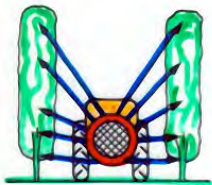
Sprühgerät mit Radialgebläse
